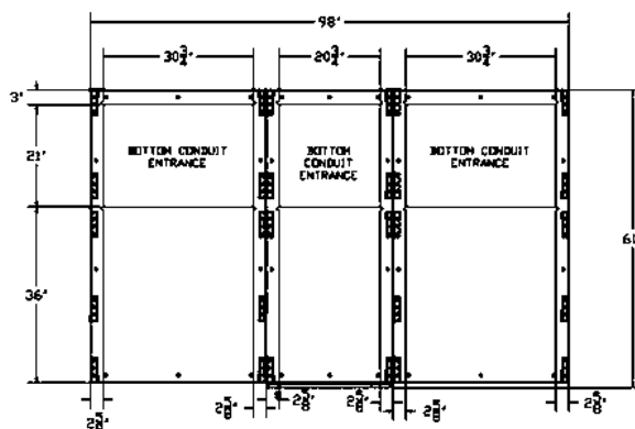
SECTION A-A (CONDUIT ENTRANCE)
