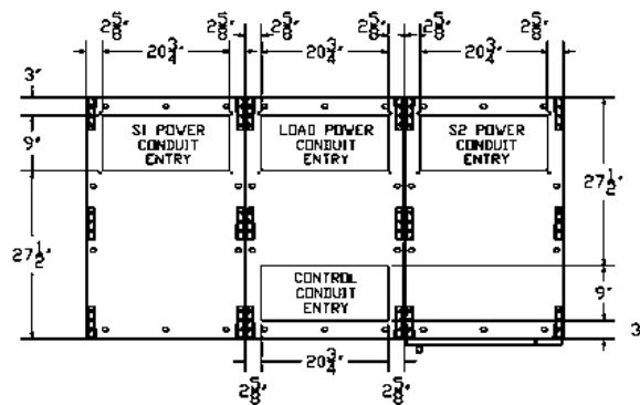
PLAN VIEW (CONDUIT ENTRY - BOTTOM)
