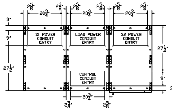
PLAN VIEW (CONDUIT ENTRY - BOTTOM)
